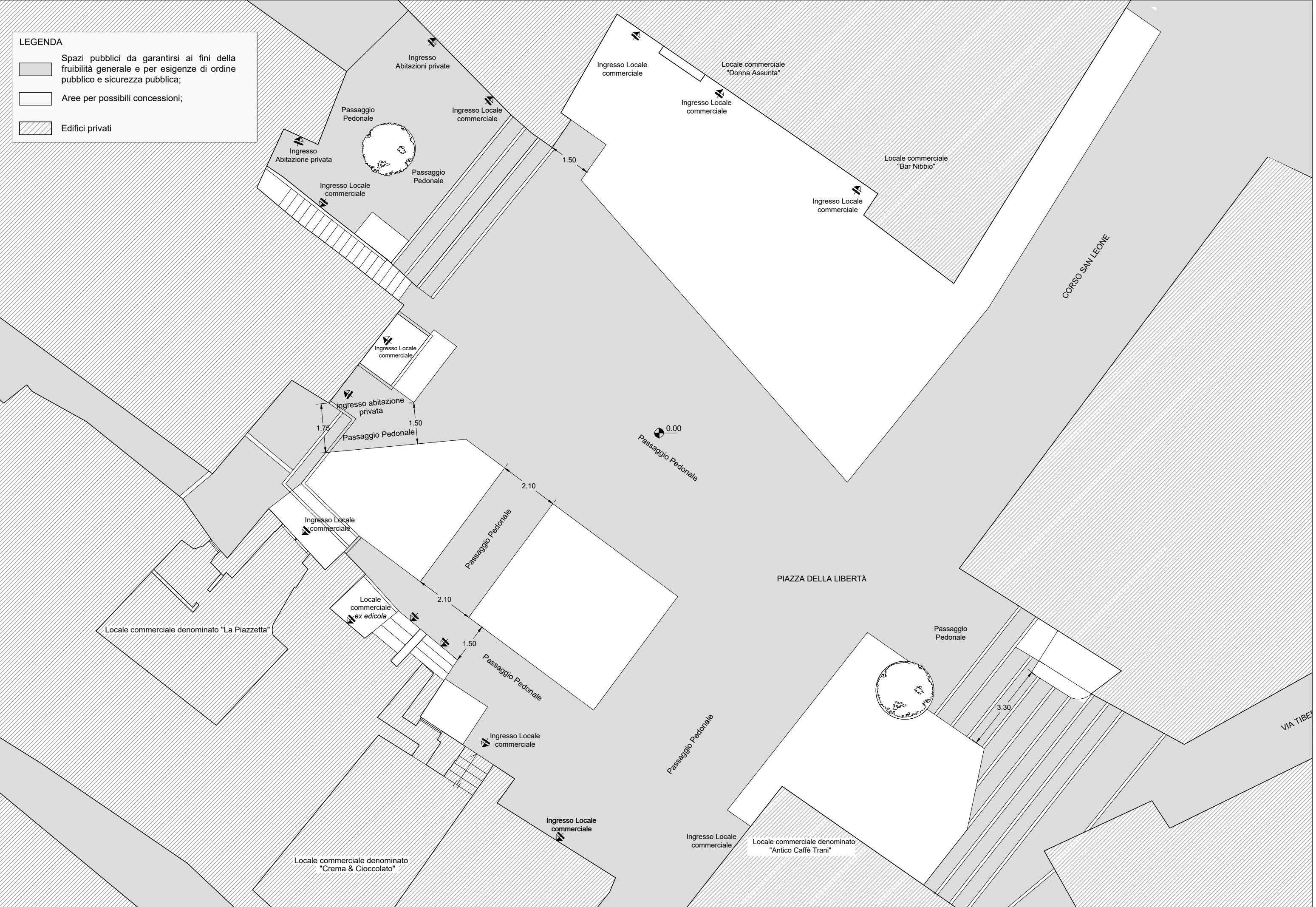
Elaborato planimetrico - Determinazione degli spazi pubblici
